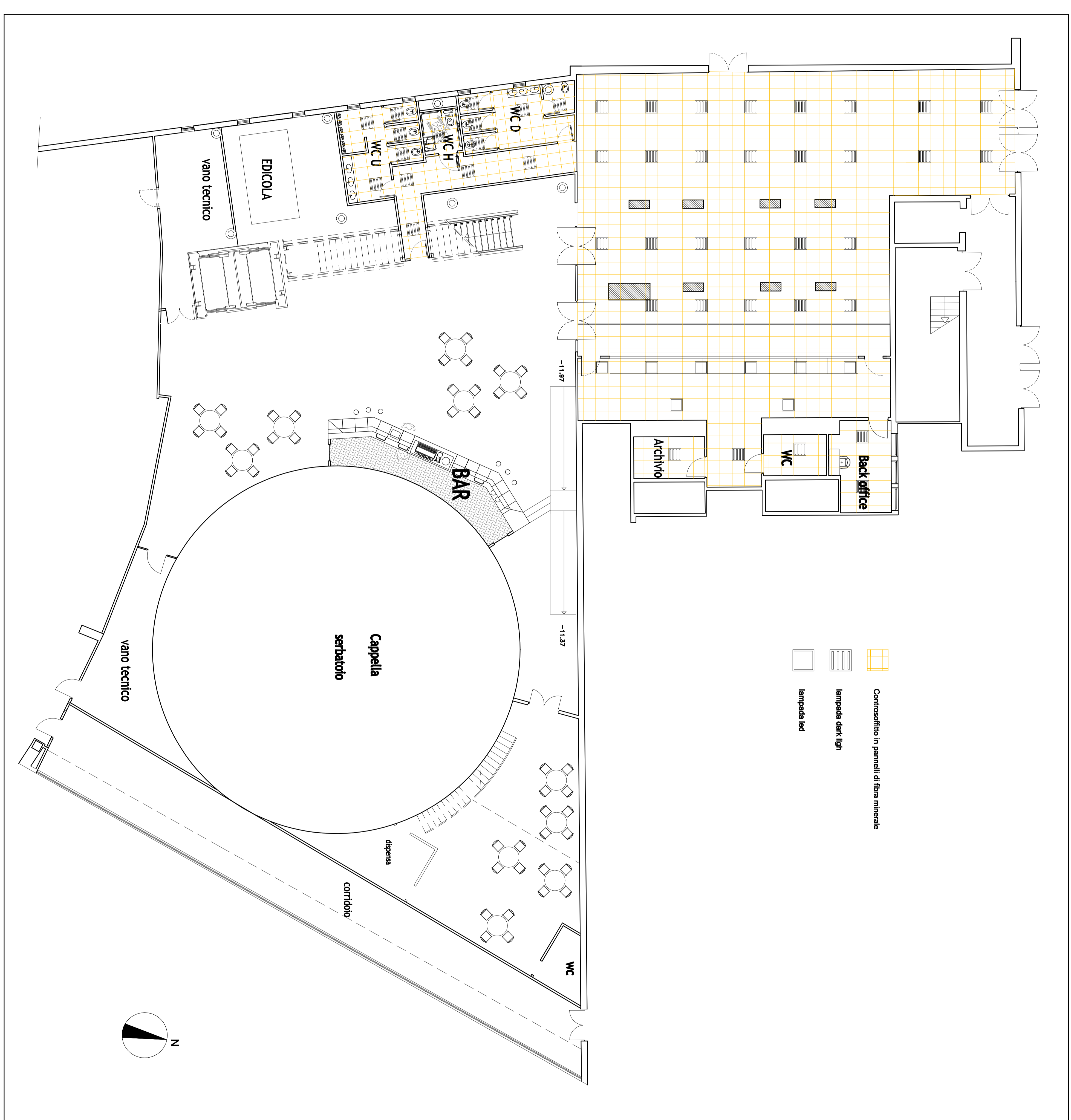
Planta CONTROSOFITTI rapp. 1:100
